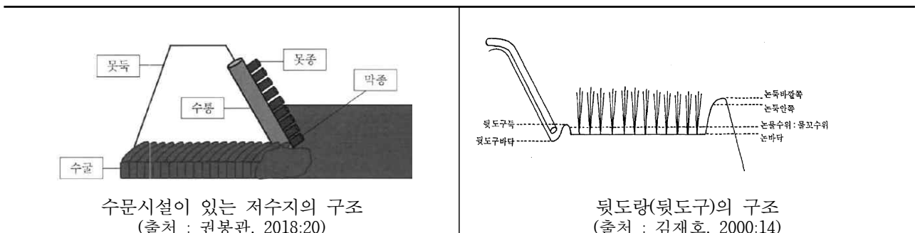
[그림 22] 저수지와 뒷도랑 구조도
