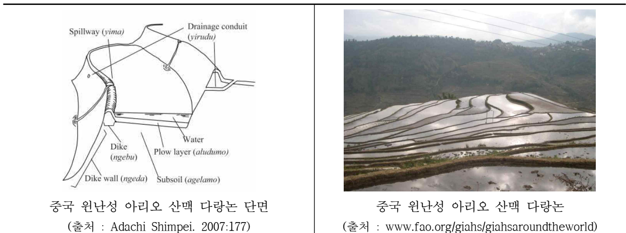
[그림 15] 점토가 발달한 지역의 다랑논 단면
